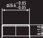
Öffnung 26,6mm Opening Ouverture
